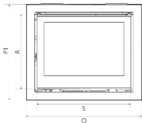
Vooraanzicht 4-zijdig kader
