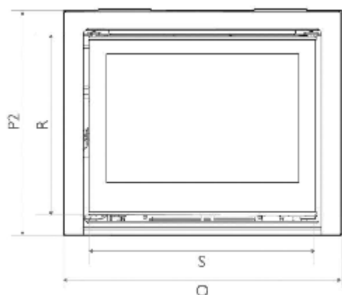
Vooraanzicht 3-zijdig kader
